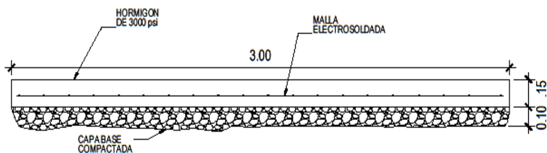
DETALLE TÍPICO DE VEREDA CALLE ESC: 1/10
