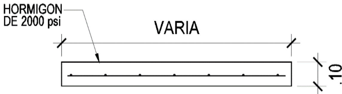
DETALLE TIPICO DE VEREDA
