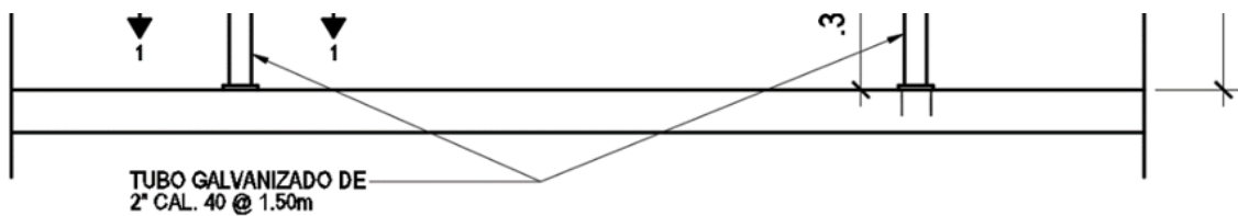
DETALLE TIPICO DE BARANDAL EN ACERA
