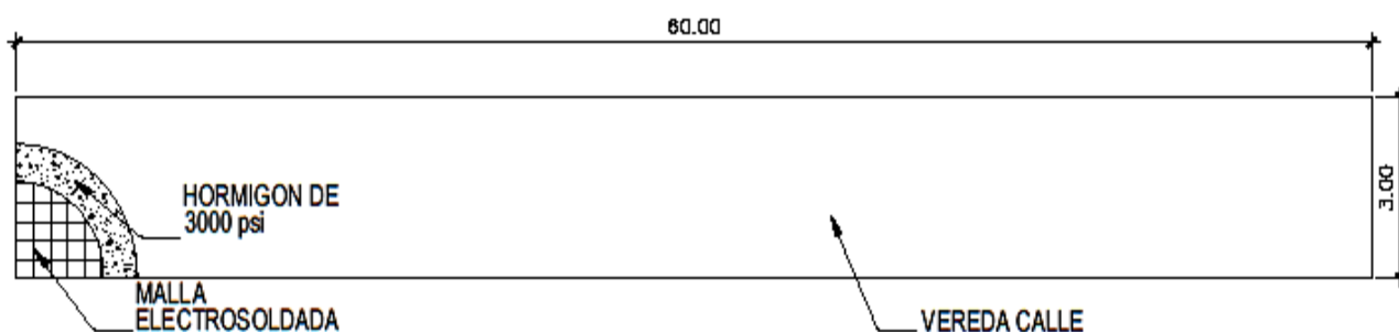
PLANTA ARQUITECTÓNICA ESC: 1/100
