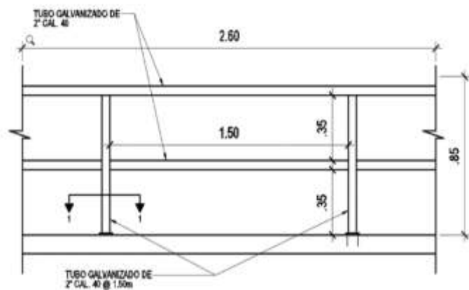
DETALLE TIPICO DE BARANDAL EN ACERA
