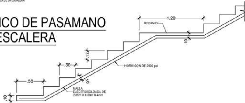
DETALLE TIPICO DE SECCION DE ESCALERA DE 1.20
