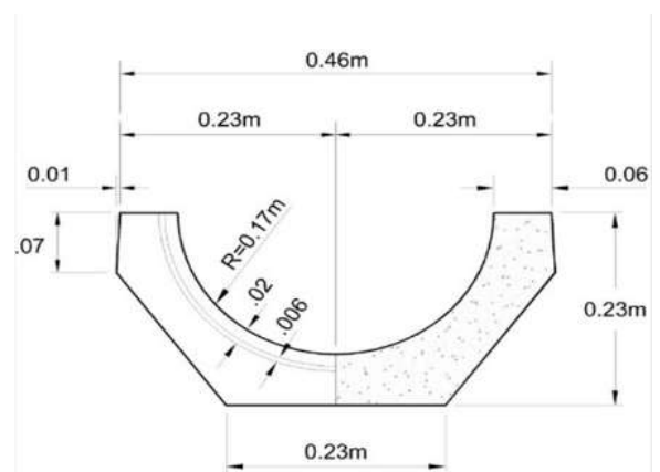
DETALLE DE MEDIA CAÑA
