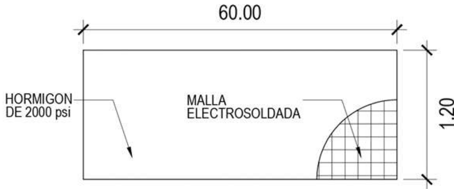
PLANTA DE VEREDA
