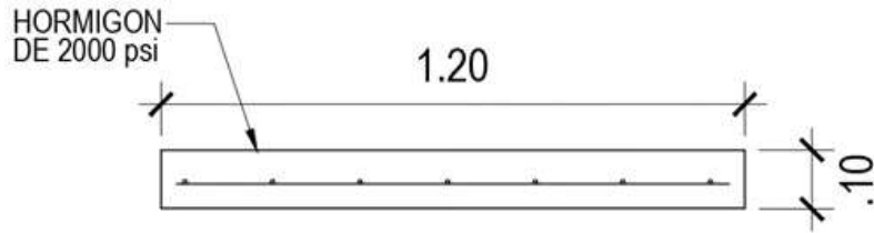
DETALLE TIPICO DE VEREDA
