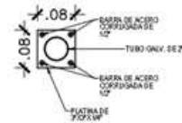
DETALLE DE ANCLAJE DE TUBO
