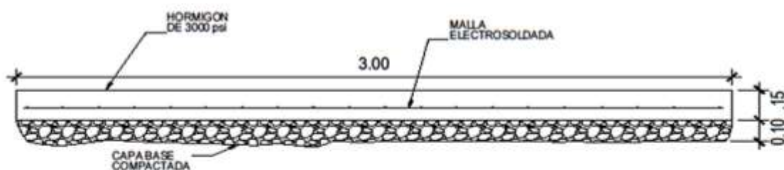
DETALLE TÍPICO DE VEREDA CALLE ESC: 1/10
