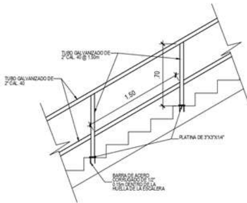
DETALLE TIPICO DE PASAMANO DE ESCALERA
