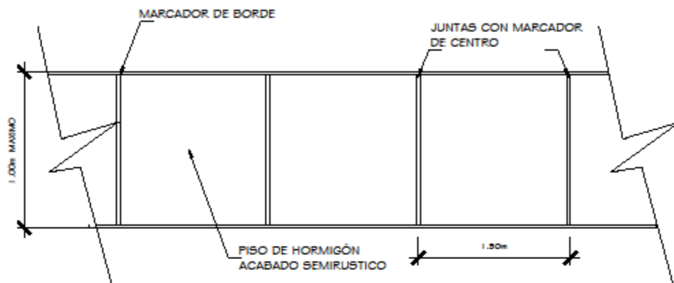
PLANTA PARCIAL DE ACERA ESC 5/E
