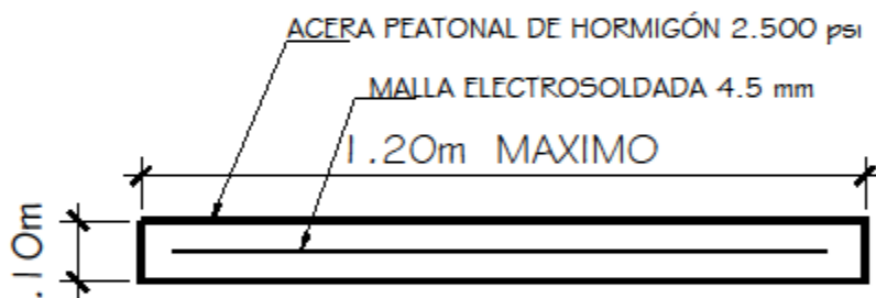
DETALLE DE ACERA ESC 1:10
