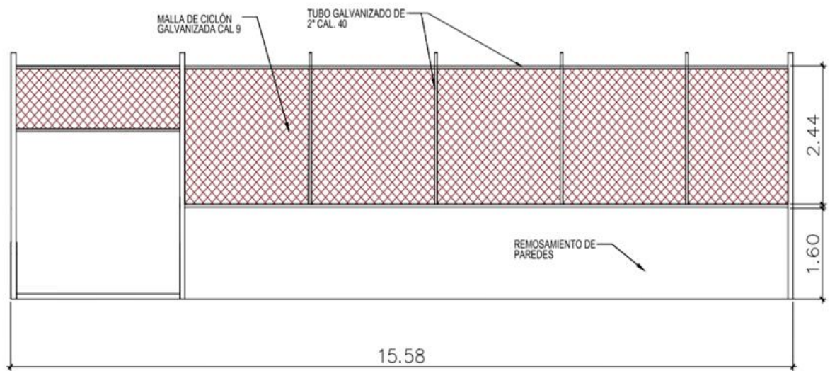
VISTA FRONTAL ESC.: S/E
