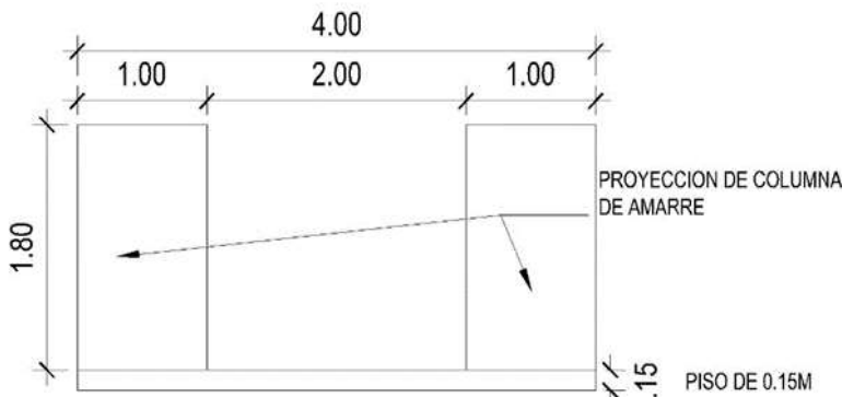
ELEVACION FRONTAL
