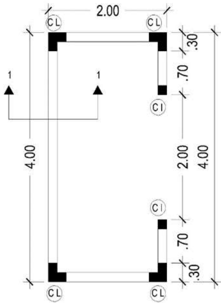
PLANTA ARQUITECTONICA
