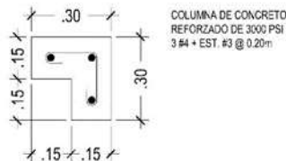
DETALLE CL
