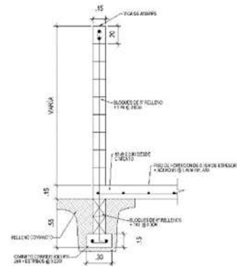
SECCIÓN 1-1
