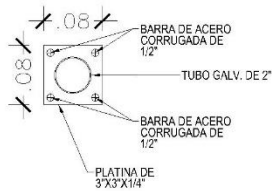
DETALLE DE ANCLAJE DE TUBO
