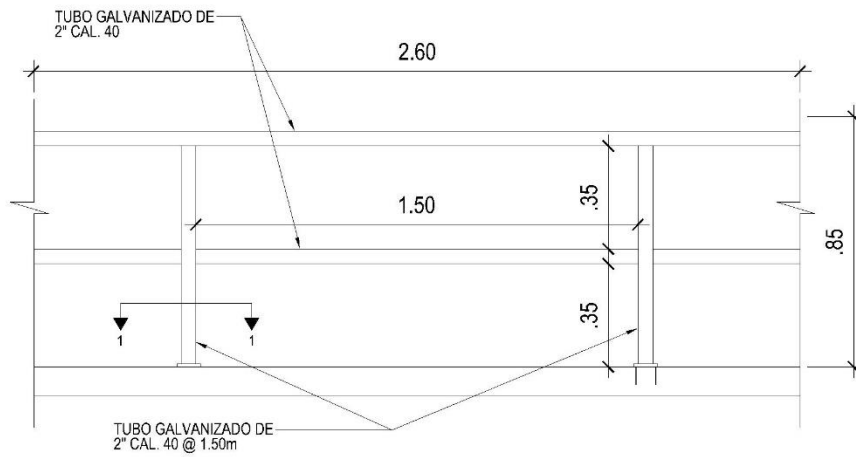
DETALLE TIPICO DE BARANDAL EN ACERA
